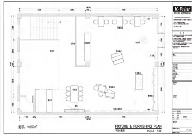
▼ 152M 2 平方平面图
