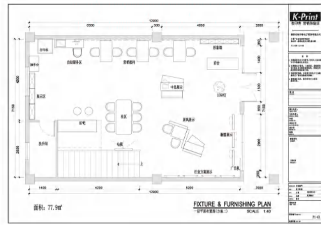
▼ 80M 2 平方平面图
